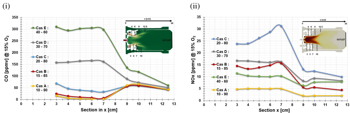
Figure 4 : Concentration croissante en CO (i) dans la chambre de combustion pilote en fonction de la distribution pilote/principal et évolution à la hausse d'émission de \text{NO}_x (ii) jusqu'à saturation (Cas C) sous l'effet d'un mélange plus riche au pilote.
