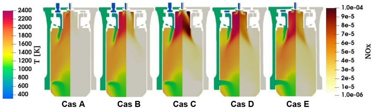
Figure 3 : Evolution du champ de température et du champ de production de \text{NO}_x où l'on voit une augmentation du niveau de températures et de \text{NO}_x jusqu'à un \Phi_{l,pilote} de 0,66 (Cas C), pour ensuite décroître légèrement.
