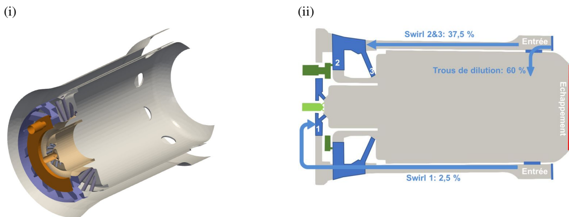
Figure 2 : Vue 3D (i) et coupe schématique de la chambre de combustion AE-T100 (ii), mettant en évidence l'arrivée d'air à contrecourant à l'extérieur de la chambre ainsi que les injecteurs de la flamme pilote (1) et de la flamme principale (2 et 3), et les trous de dilution.
