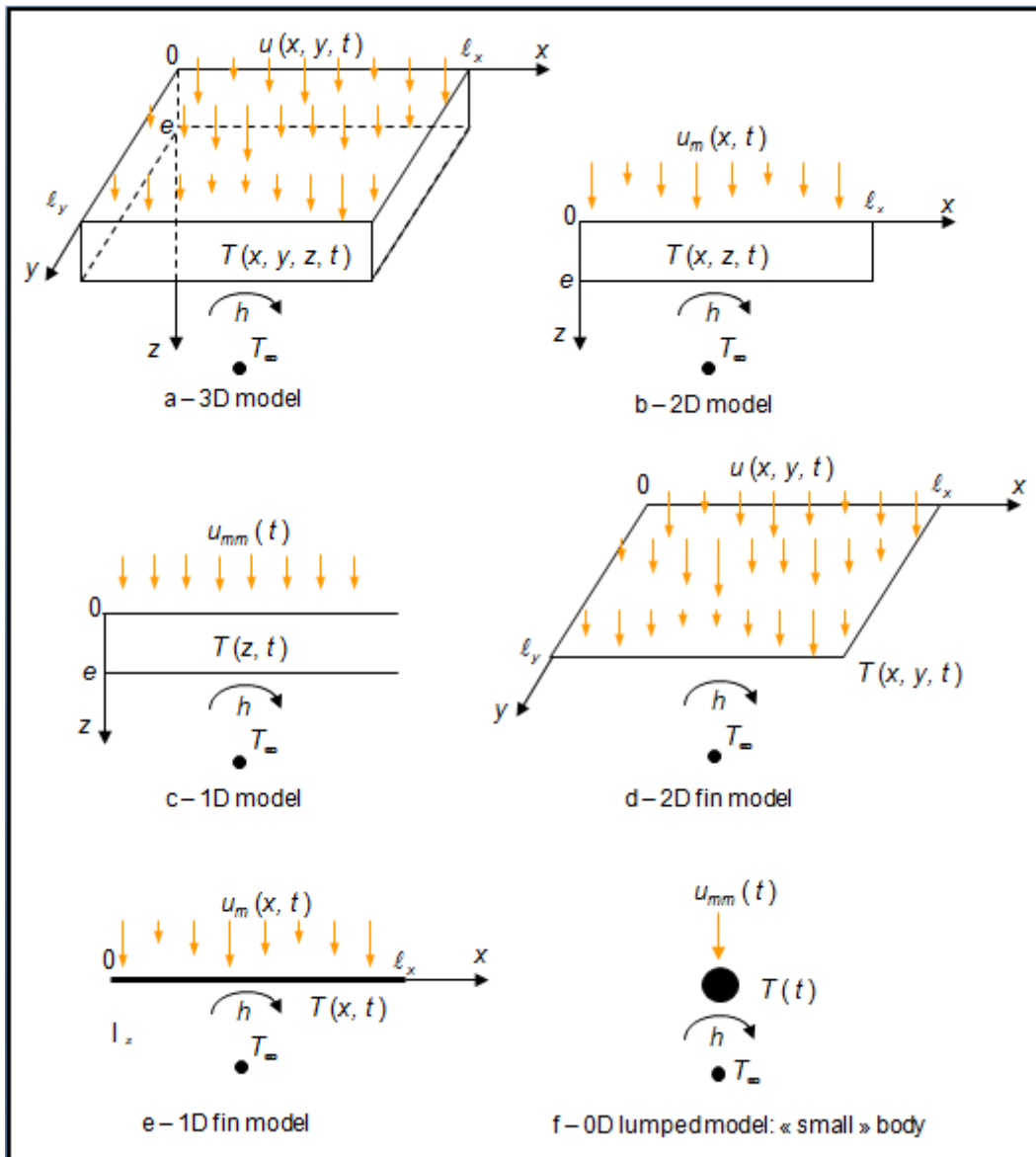
Figure 9. « Physical » model reduction
